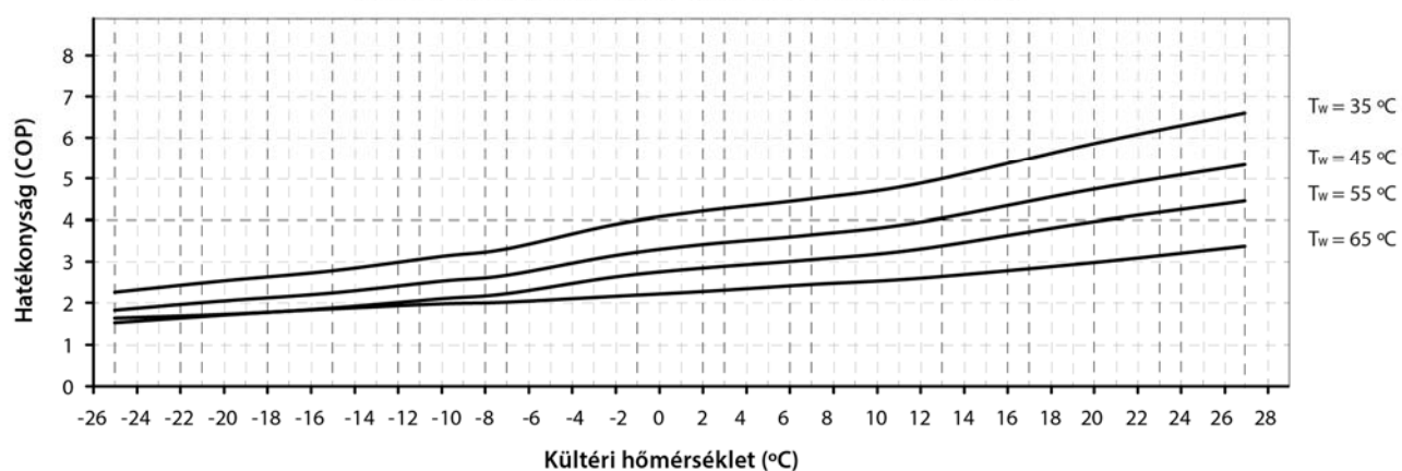
Fűtési hatékonysági görbék Dual Clima 12HT/12HTT (COP)
