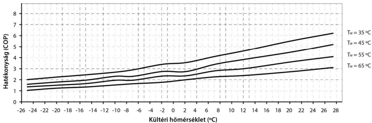
Fűtési hatékonysági görbék Dual Clima 22HTT (COP)
