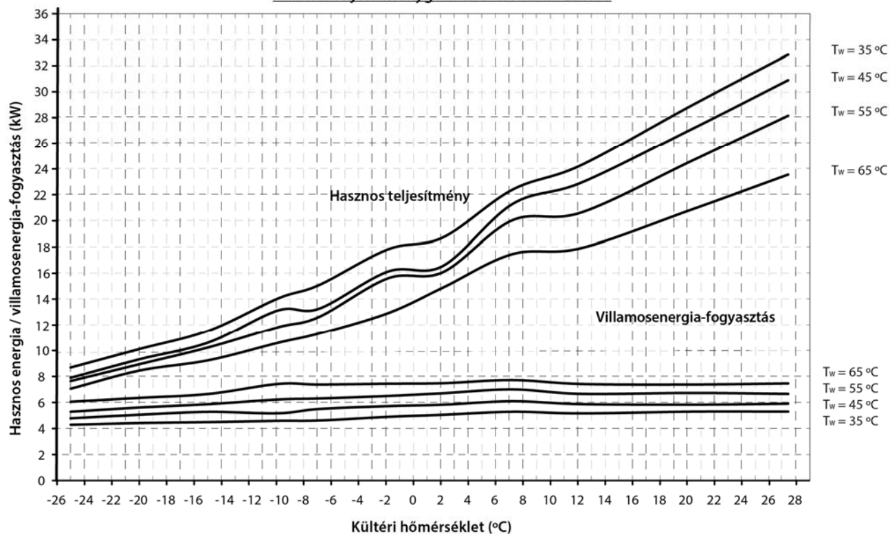
A fűtési teljesítménygörbék Dual Clima 22HTT
