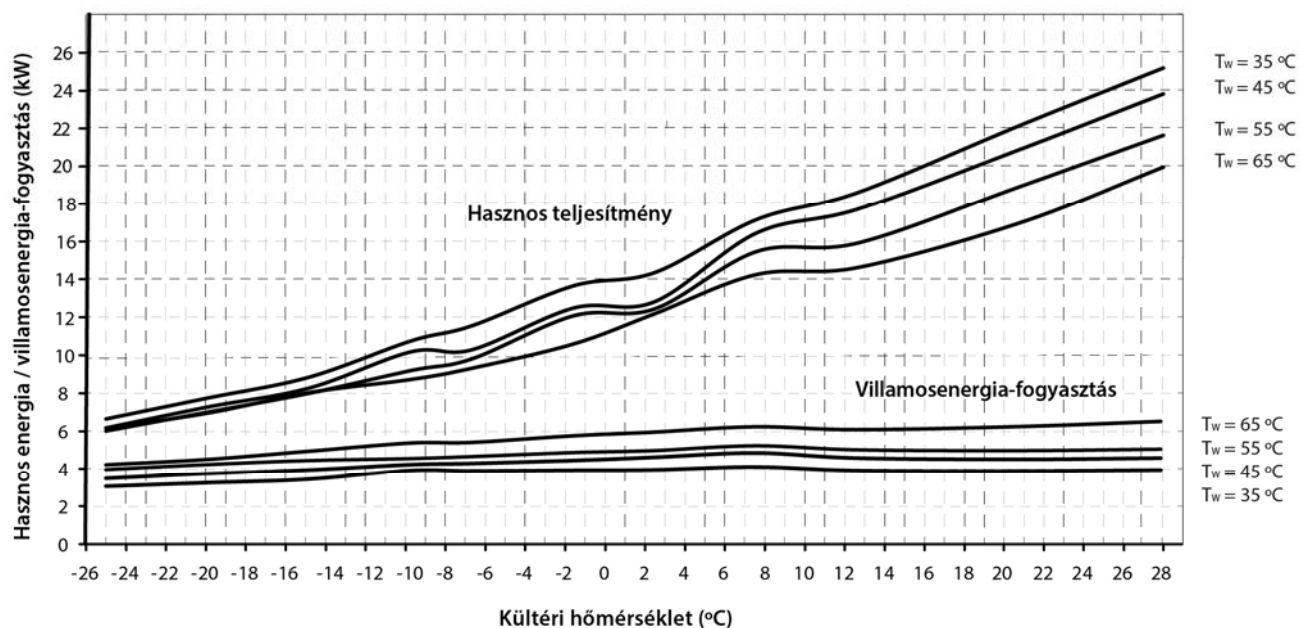
A fűtési teljesítménygörbék Dual Clima 16HT/16HTT
