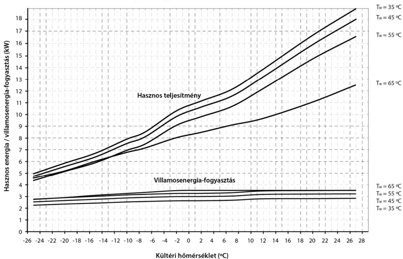
A fűtési teljesítménygörbék Dual Clima 12HT/12HTT
