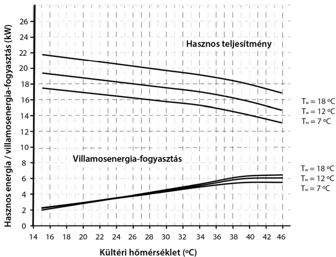
Kettős Clima 19HT/19HTT hűtési teljesítménygörbék
