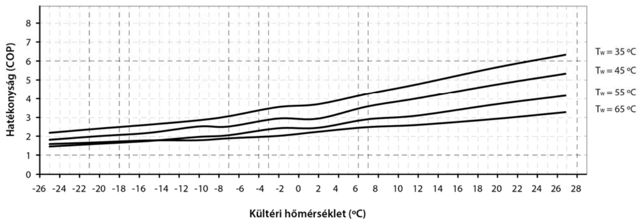
Fűtési hatékonysági görbék Dual Clima 16HT/16HTT (COP)
