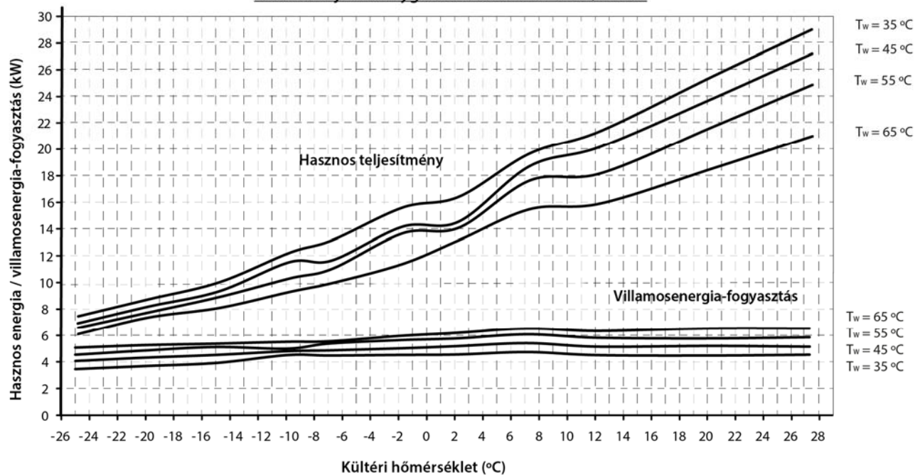
A fűtési teljesítménygörbék Dual Clima 19HT/19HTT
