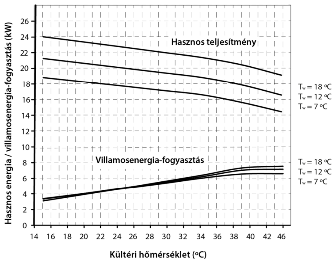
Kettős Clima 22HTT hűtési teljesítménygörbék
