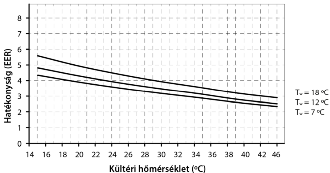
Dual Clima 19HT/19HTT hűtési hatékonysági görbék (EER)
