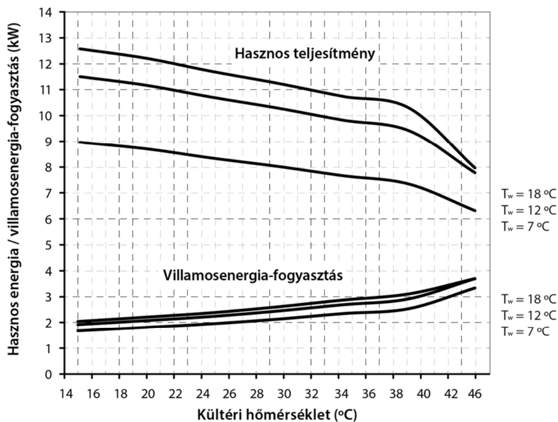
Kettős Clima 12HT/12HTT hűtési teljesítménygörbék
