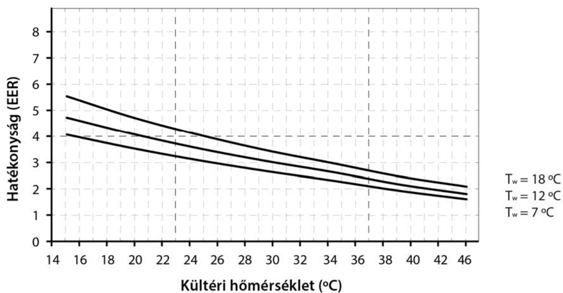
Dual Clima 22HTT hűtési hatékonysági görbék (EER)
