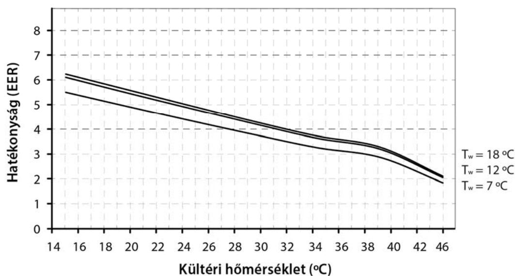
Dual Clima 12HT/12HTT hűtési hatékonysági görbék (EER)
