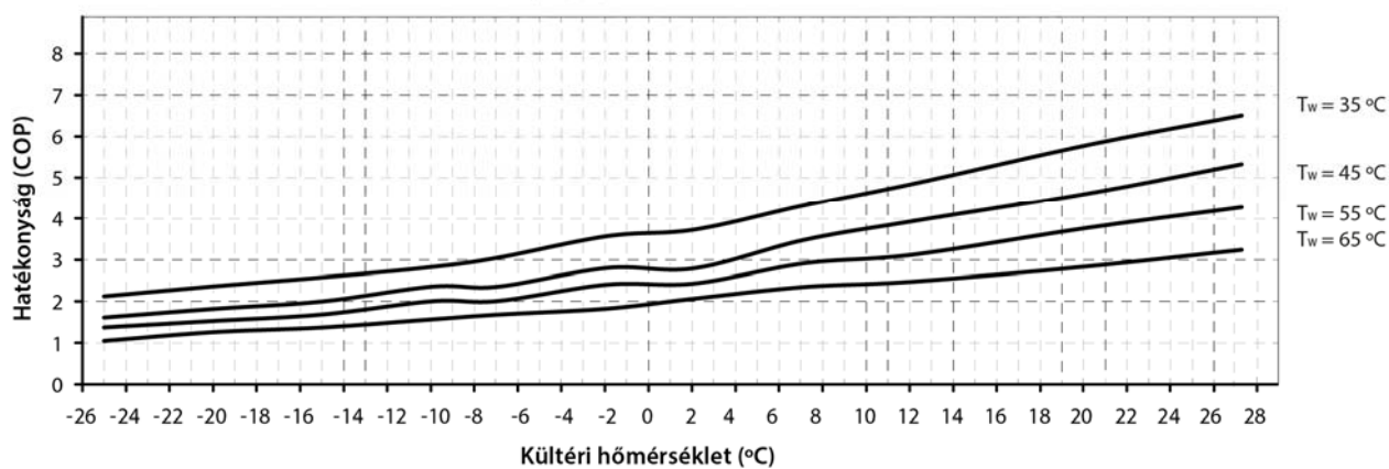
Fűtési hatékonysági görbék Dual Clima 19HT/19HTT (COP)
